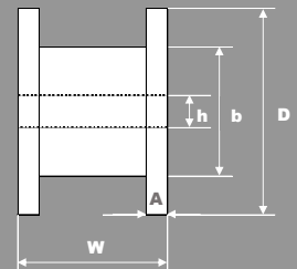
ポピン形状
